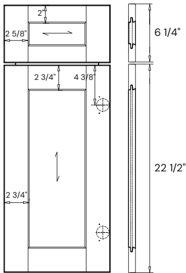
Door Profile
